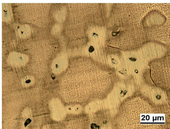
Fig. 1 - Microstruttura del bronzo (attacco metallografico con soluzione di \text{FeCl}_3 , osservazione al microscopio ottico). Bronze microstructure (metallographic attack by \text{FeCl}_3 solution, optical microscope observation).
