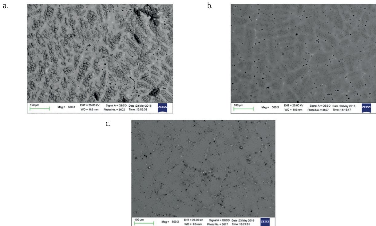
Fig. 3 - Immagini al SEM ottenute con elettroni retrodiffusi su campioni di bronzo dopo immersioni in ARX10, sia in assenza di inibitori (a) che in presenza di SITP (b) o SITP+P (c). SEM images obtained with backscattered electrons on bronze samples after exposure to ARX10, both in the absence (a) and in the presence of SITP (b) or SITP + P (c).
