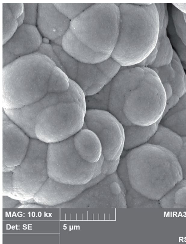
Fig. 6 - Immagine SEM del palladio ottenuto con deposizione electroless.
