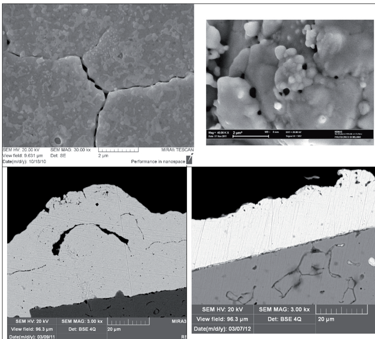
Fig. 11 - Morfologia delle due membrane esercite: a) V3 e b) V2
