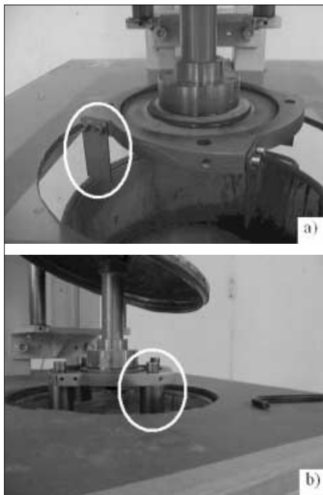
Fig. 1 – Vista dell'apparato di idroerosione con campioni a) piatti e b) cilindrici montati.
