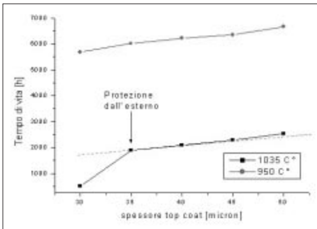
Fig. 10 – Andamento del tempo di vita in funzione dello spessore del top coat per il rivestimento duplex.
