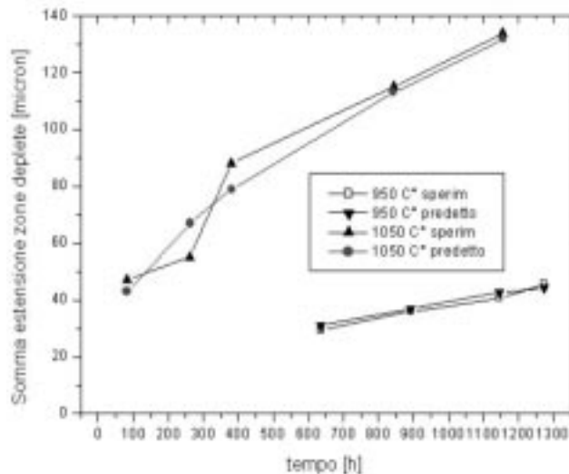
Fig. 5 – Zone deplete di un rivestimento di AMDRY 995, dopo ciclaggio termico a 1050°C – 600 cicli di un’ora (a sinistra). Accordo tra valori della somma delle due zone deplete previsti dal modello e misurati su campioni di prove di laboratorio (a destra).
